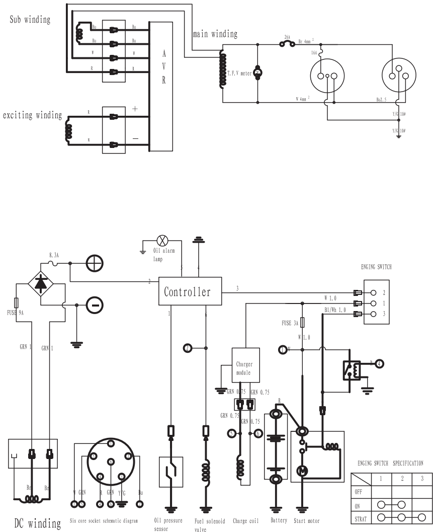
Figura 5-1 diagrama del circuito de tensión única monofásico
