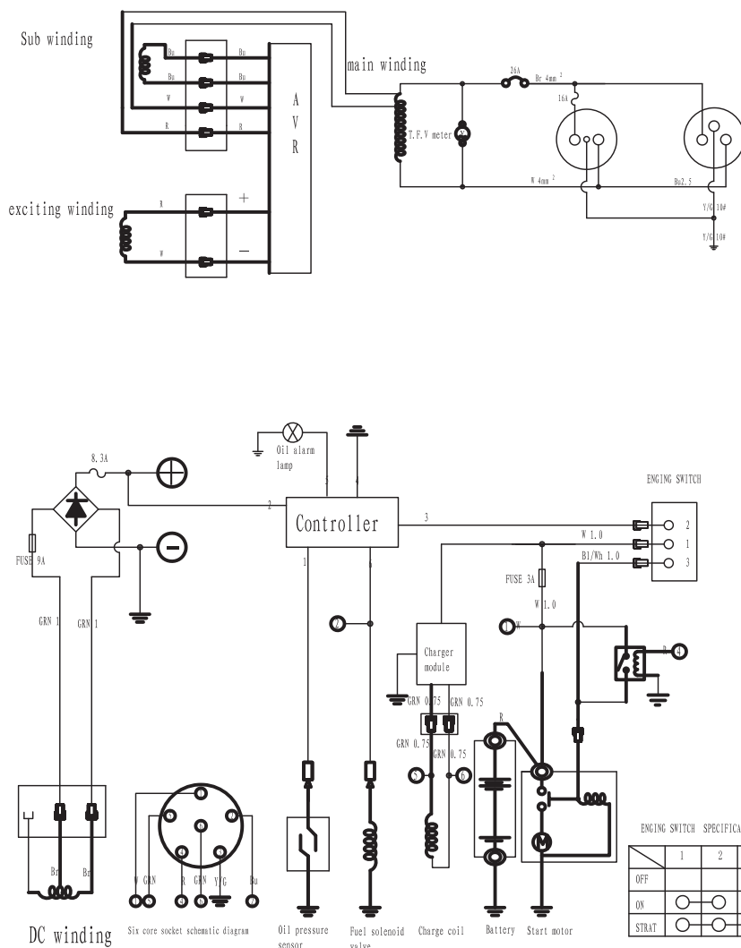
Figura 5-1 diagramma di circuito a singolo voltaggio monofase
