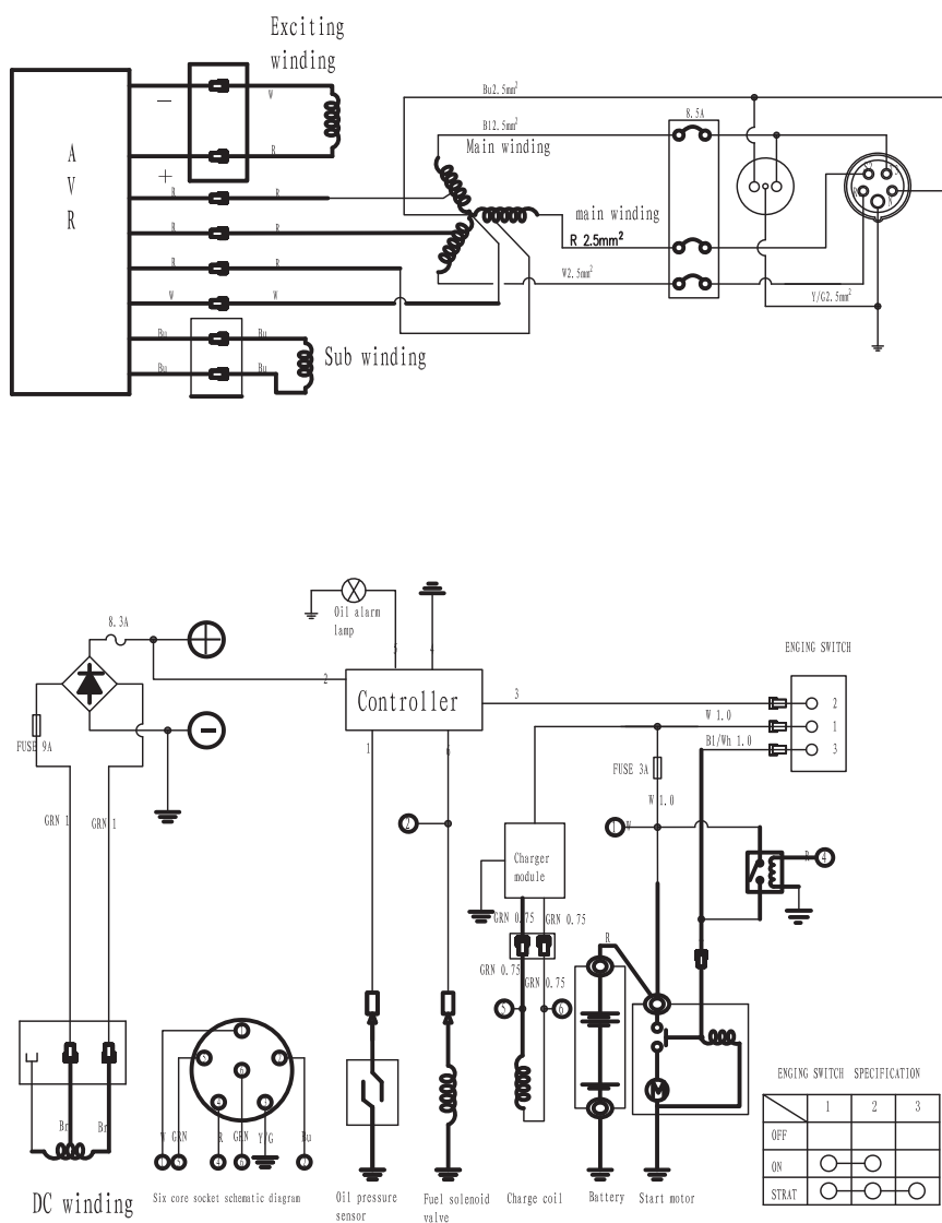
Figura 5-2 diagramma di circuito trifase
